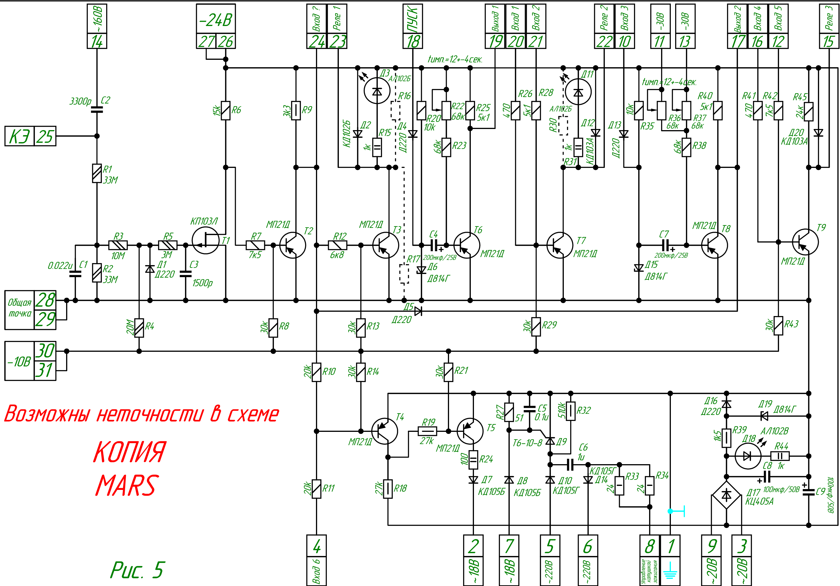
Принципиальная схема субблока Ф-04
