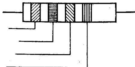
Рис. 1. Маркировка резистора с номинальным сопротивлением 47 кОм и допуском \pm 5\%
